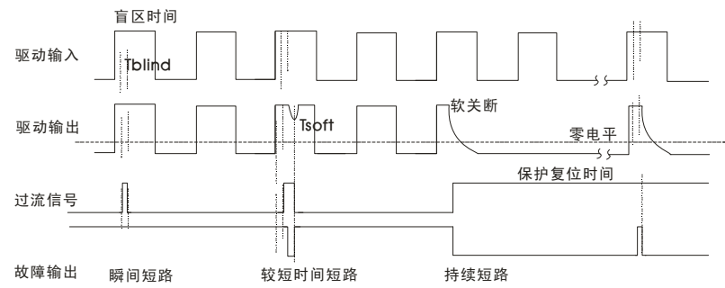
图 2 保护示意图
