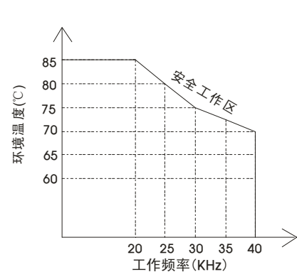
图 4 QC962-8A 安全工作区
