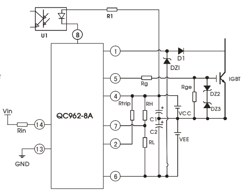
图9 减小保护抑制时间
