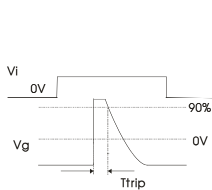
图7 保护抑制时间测试
