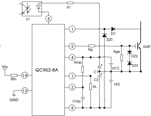
图 6 增加保护阈值电压
