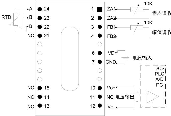
图 3 电压输出型产品应用接线图
