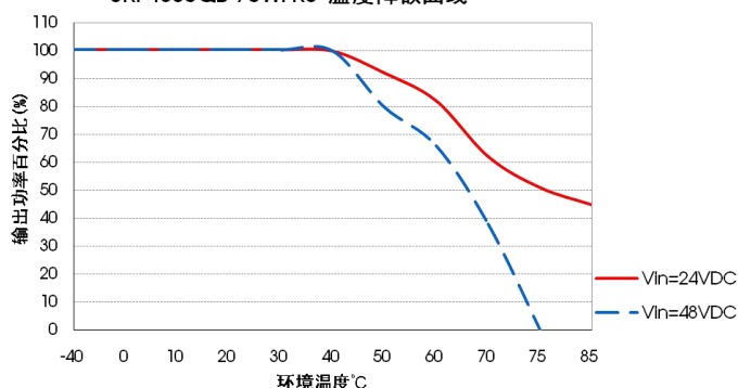
URF4805QB-75WFR3 温度降额曲线
