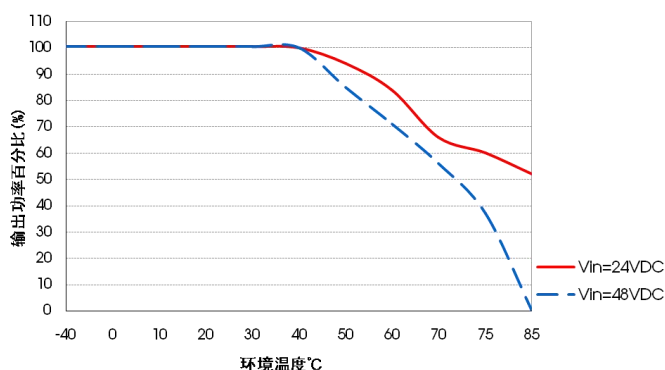
URF4805QB-75WHR3 温度降额曲线
