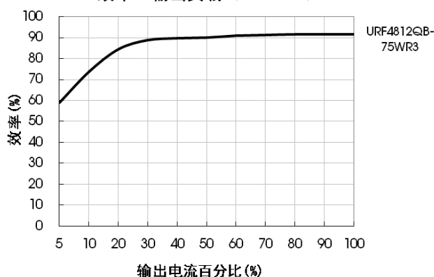
效率Vs输出负载 ( V_{in}=48\text{V} )
